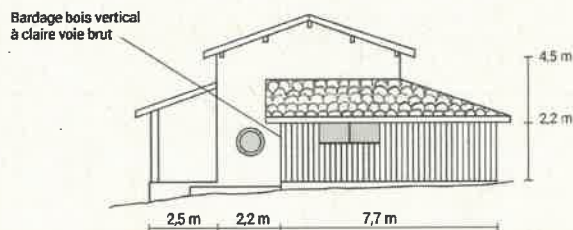
FAÇADE EST
