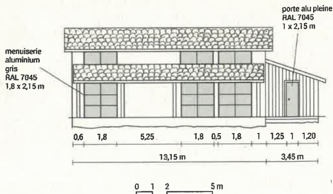
FAÇADE SUD
