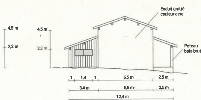
FAÇADE OUEST
